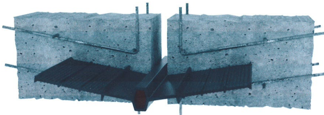
Innenliegendes Dehnfugenband
